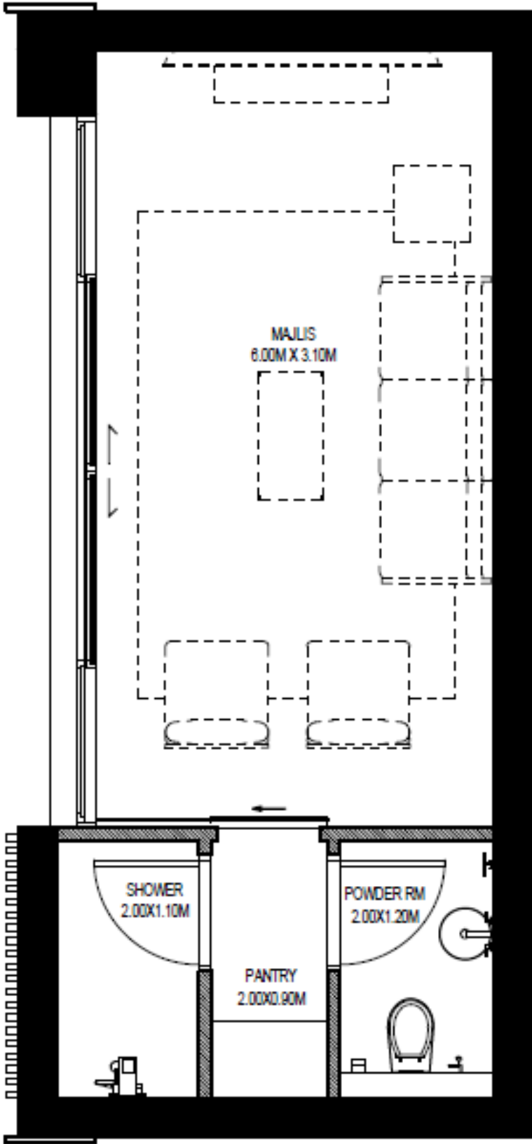
MAJLIS LAYOUT
